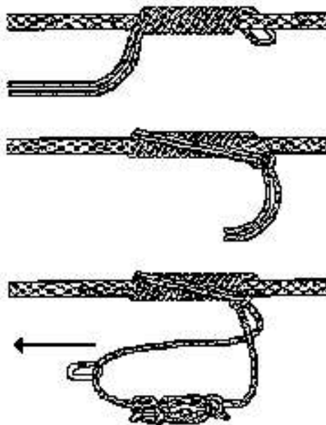
KLEIMHEIST
